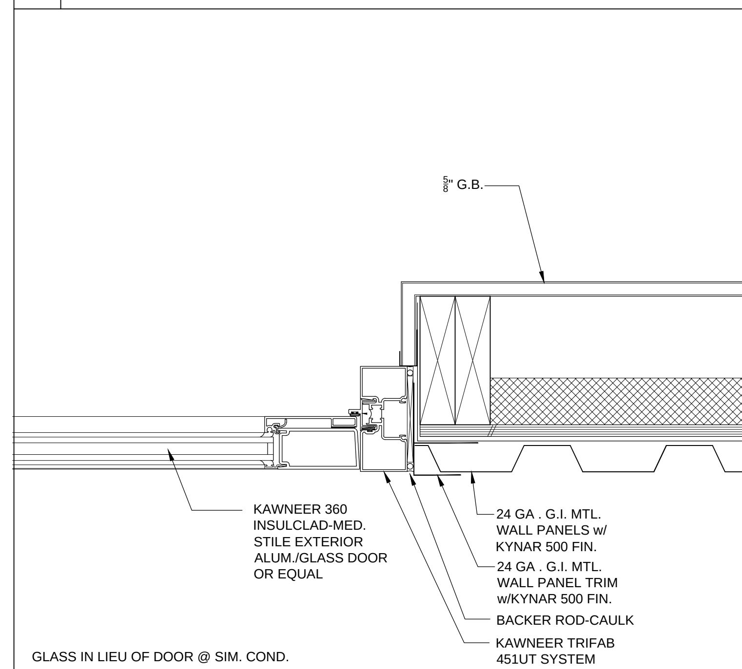
8 JAMB DETAIL
