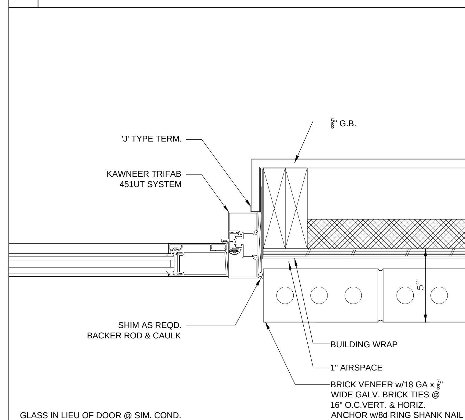
4 JAMB DETAIL
