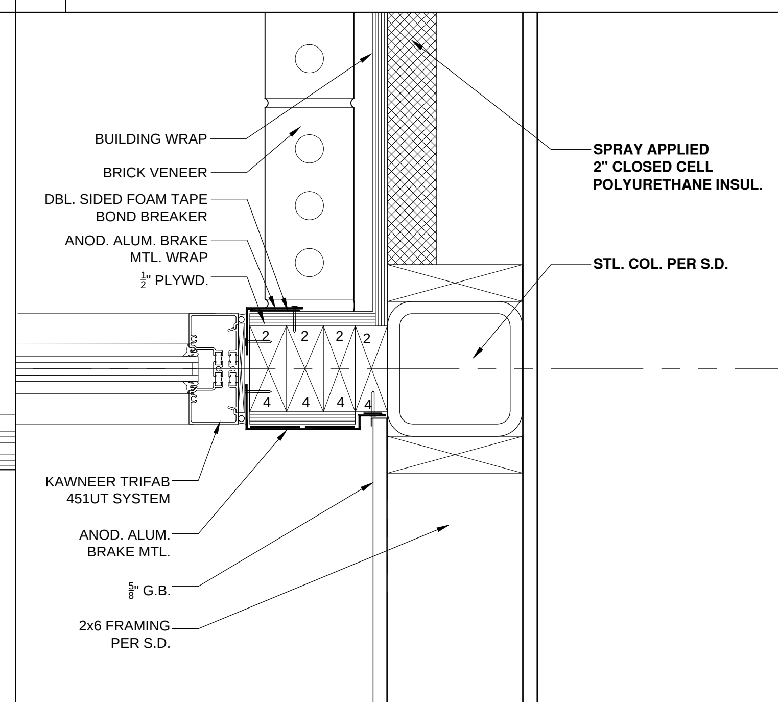
2 JAMB DETAIL
