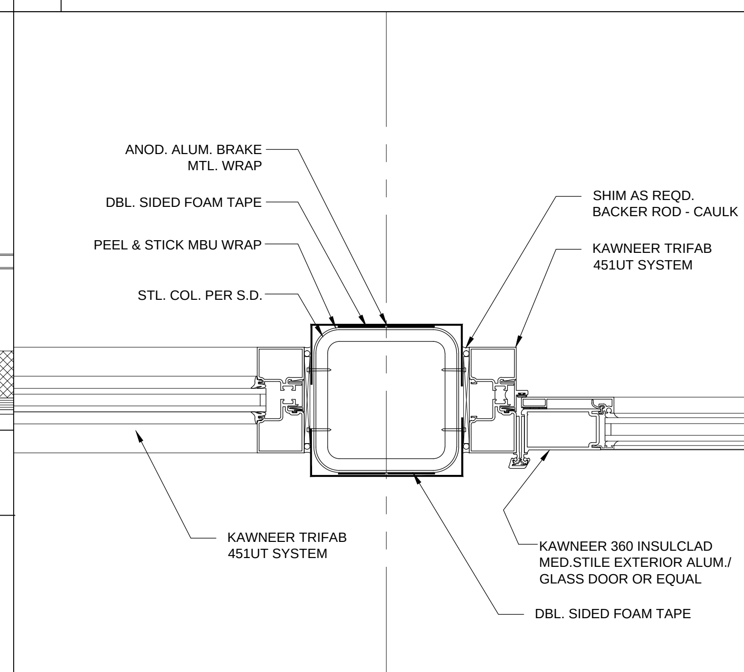
3 JAMB DETAIL
