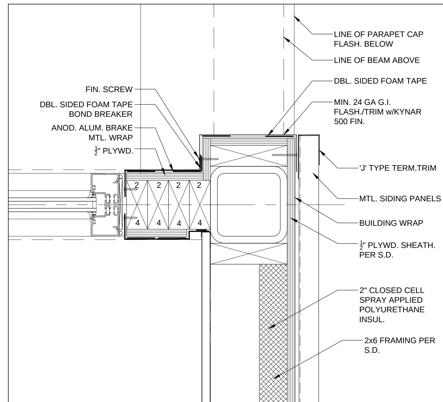
12 JAMB DETAIL
