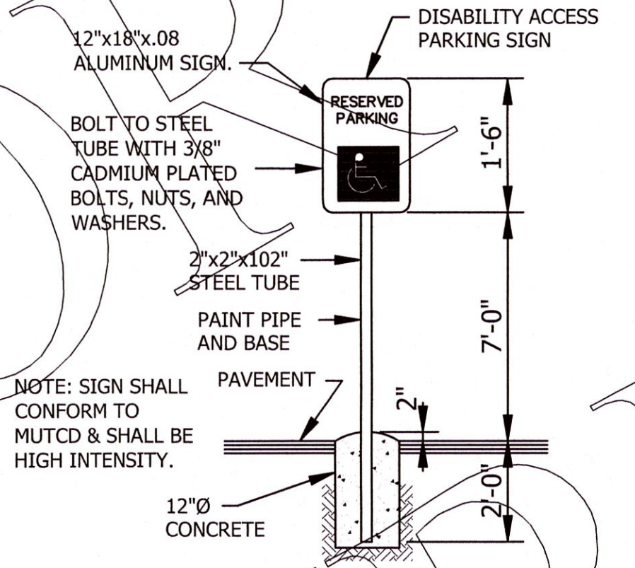
ADA SIGN DETAIL N.T.S.
