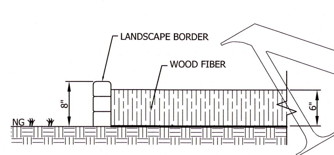
SECTION 'B-B' (NIC) N.T.S.
