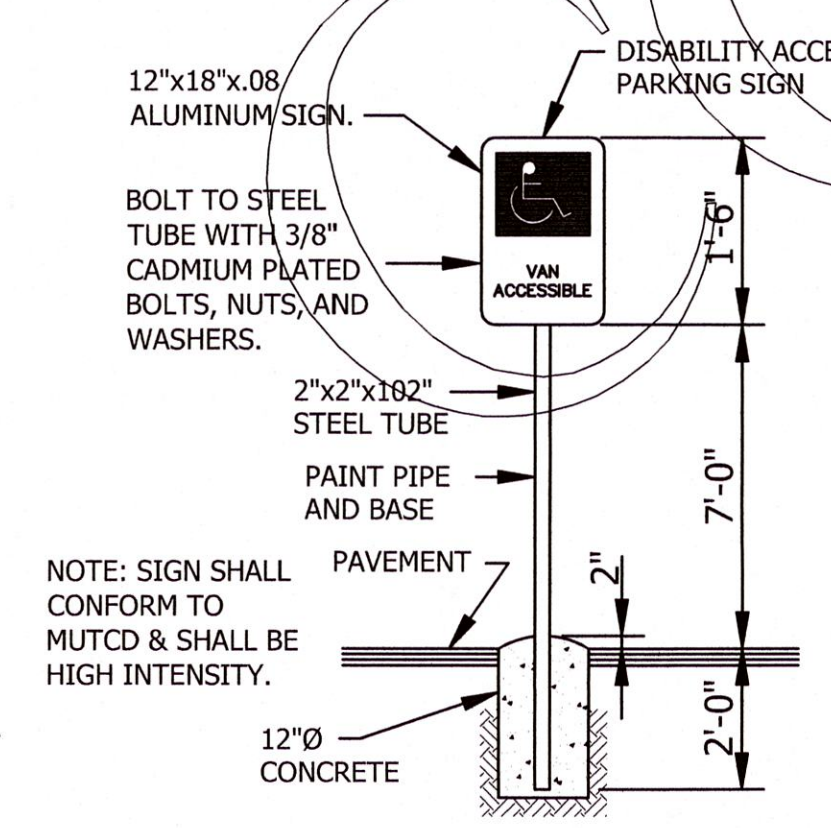
ADA VAN ACCESSIBLE SIGN DETAIL N.T.S.
